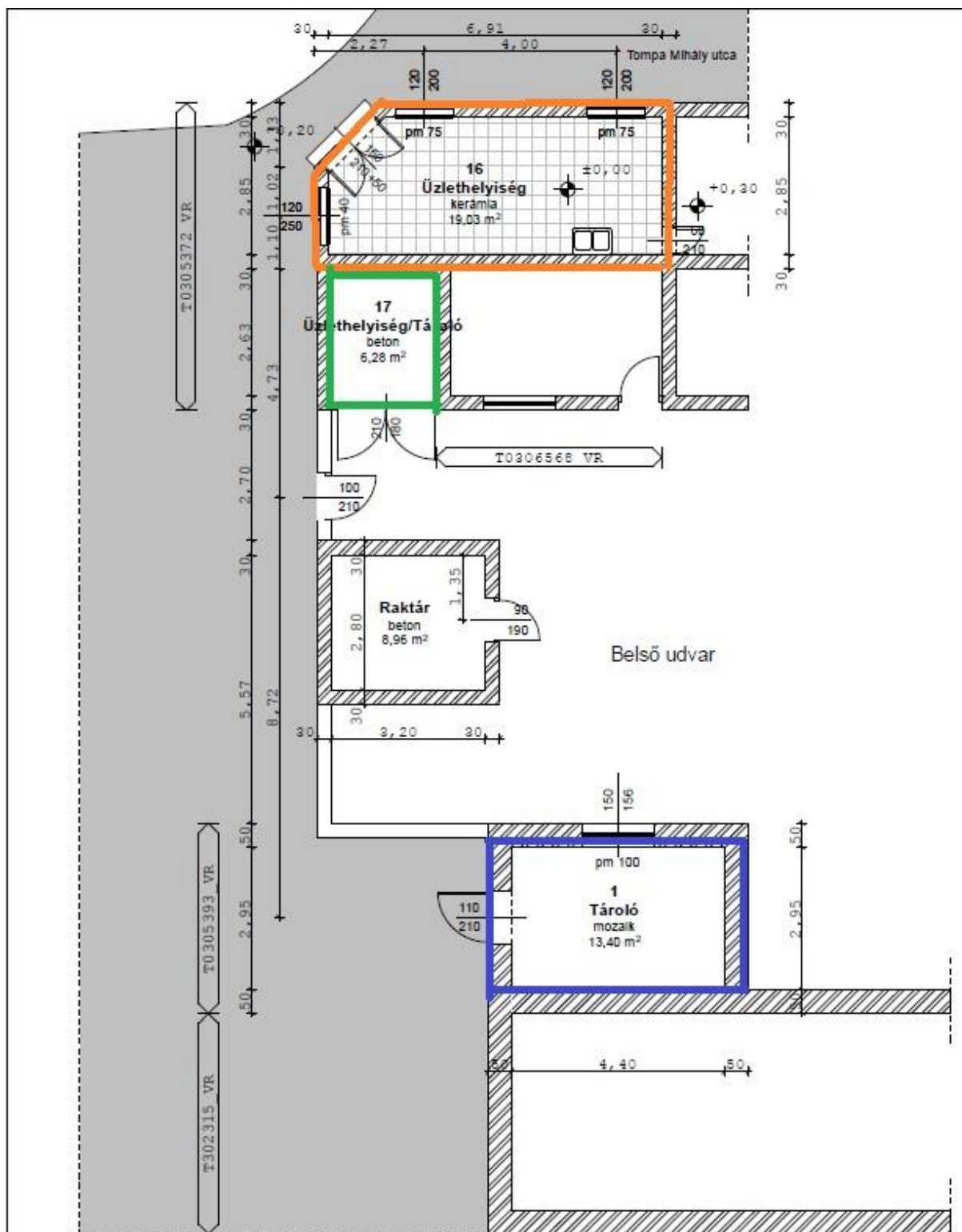
Földszinti alaprajz M 1:100
